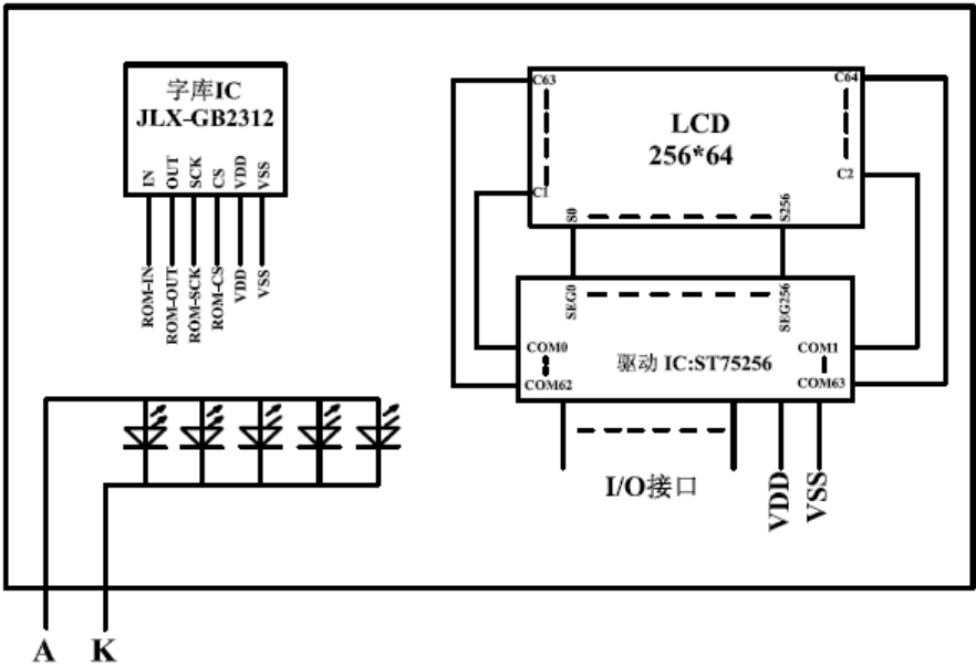
图 2: JLX25664G-251-PC 电路框图
