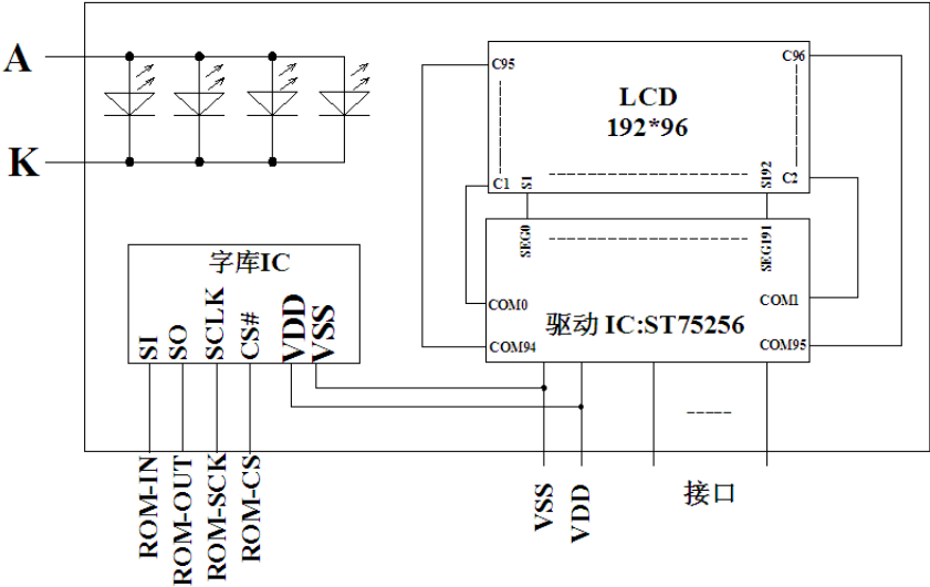
图 2：JLX19296G-919-PL 电路框图
