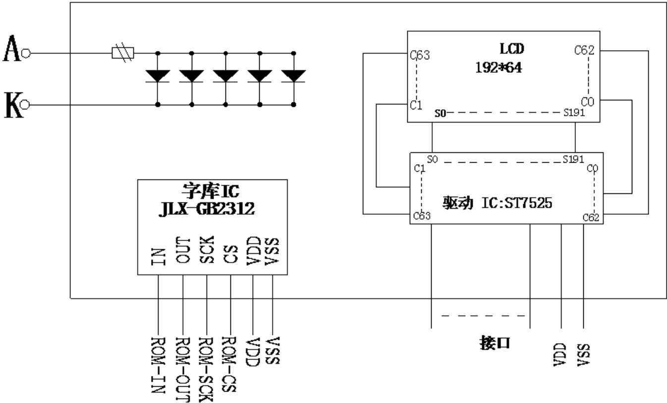
图 2: 电路框图
