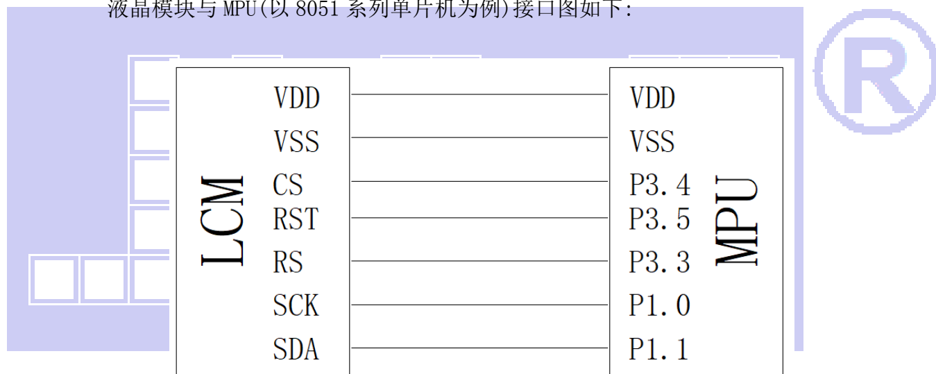
图 9. 串行接口
