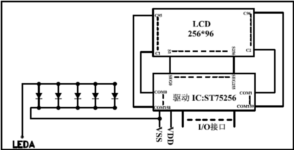
图 2：JLX25696G-968-PN 图像点阵型液晶模块的电路框图
