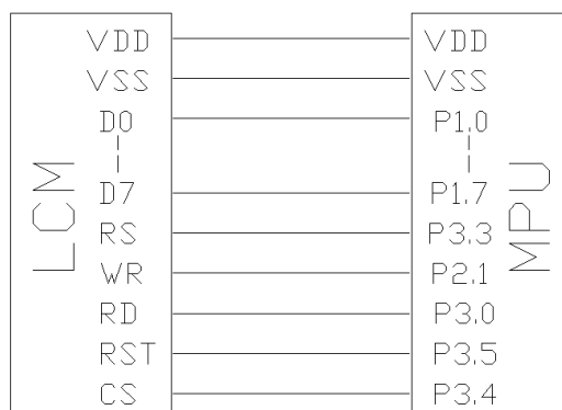
图 8: 并行接口图
