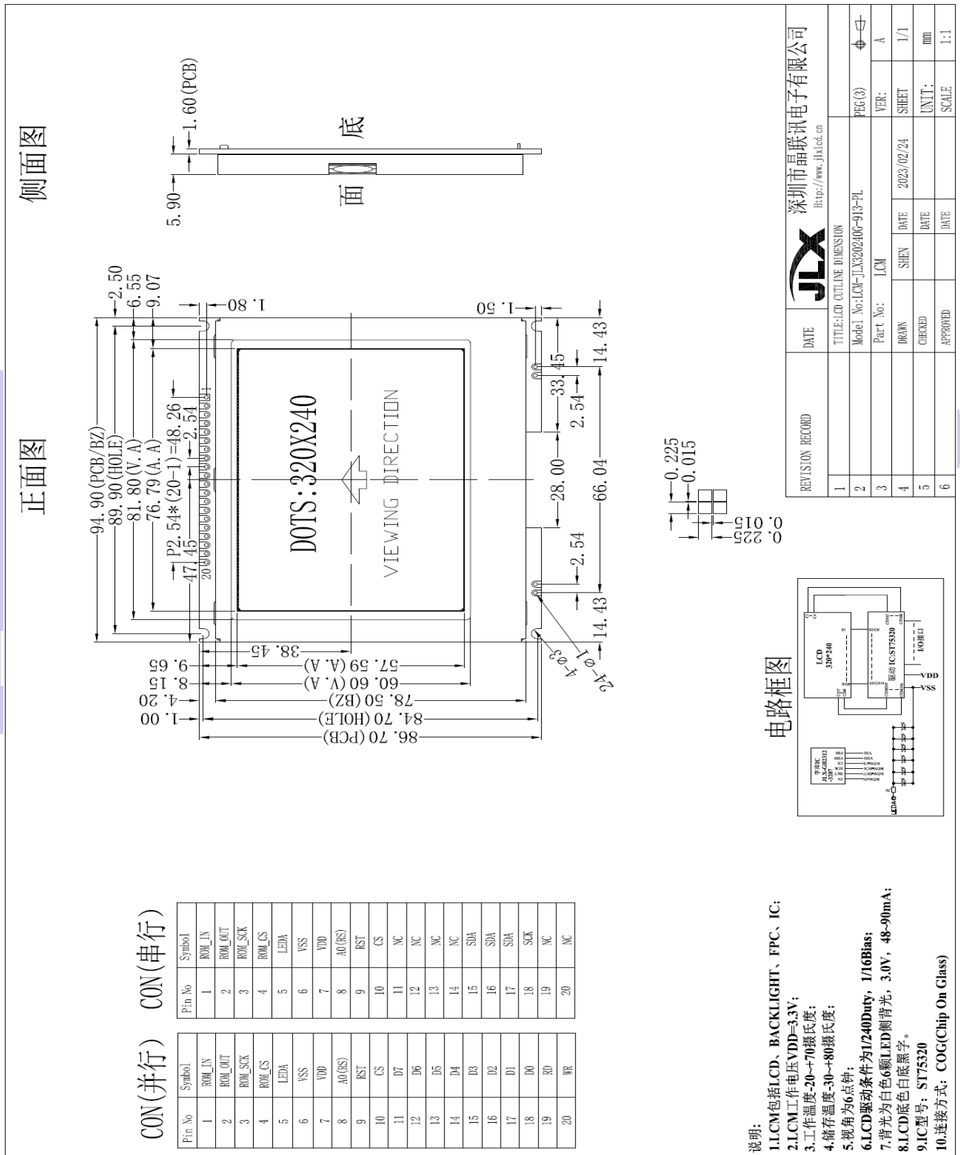
图 1. 外形尺寸
