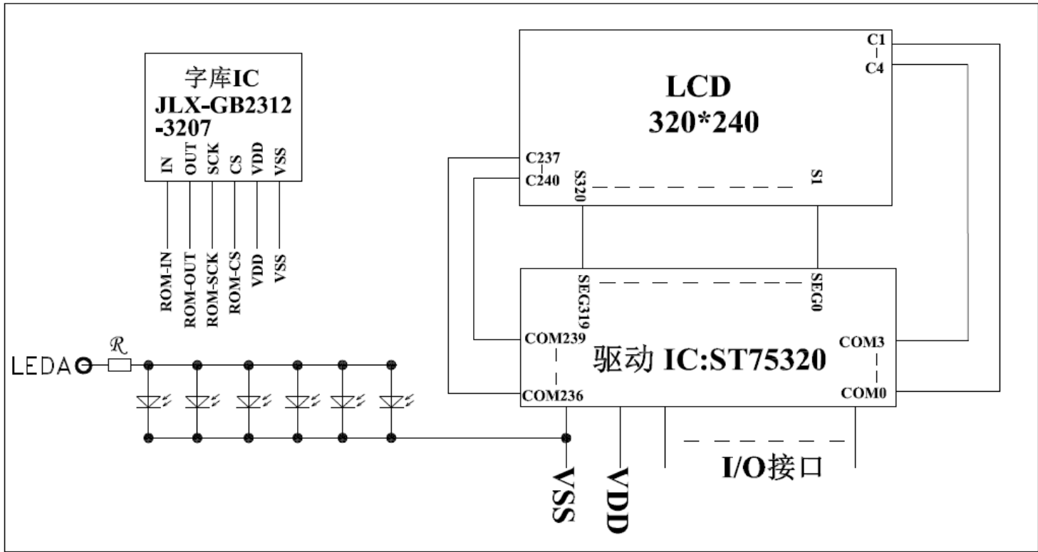
图 2: JLX320240G-913-PL 电路框图
