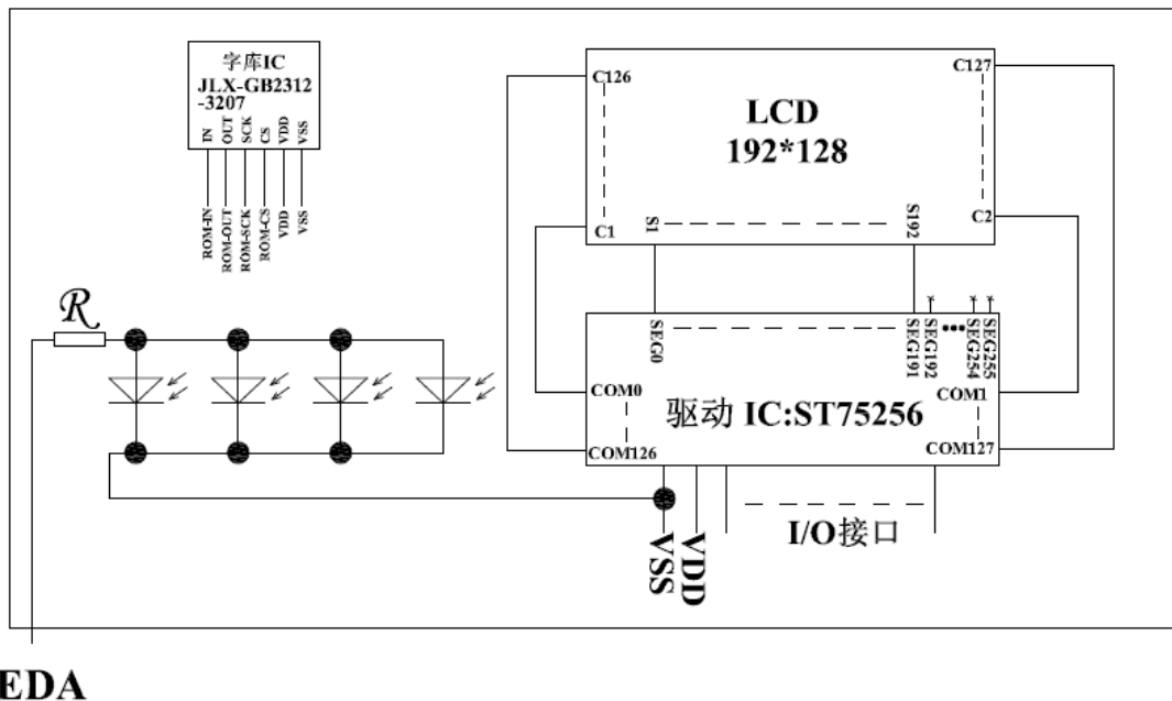
图 2: JLX192128G-970-PL 电路框图
